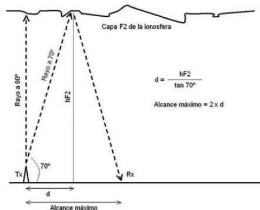
Figura 1: esquema de un enlace de radio por NVIS
