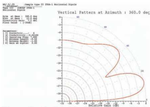
Figura 5: dipolo ubicado a una longitud de onda del suelo
