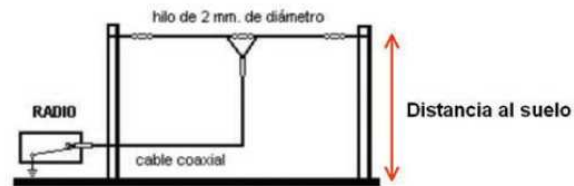
Figura 4: dipolo de hilo horizontal
