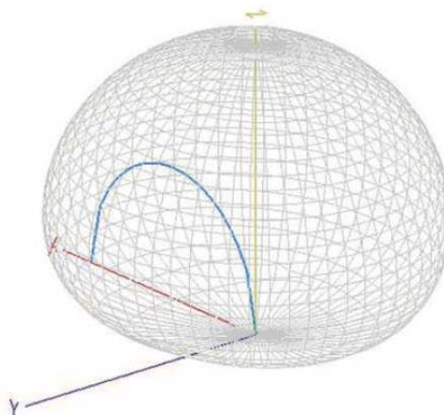
Figura 9: diagrama de radiación de una antena NVIS de medio bucle
