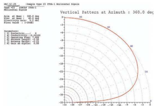
Figura 6: dipolo ubicado a un cuarto de longitud de onda del suelo
