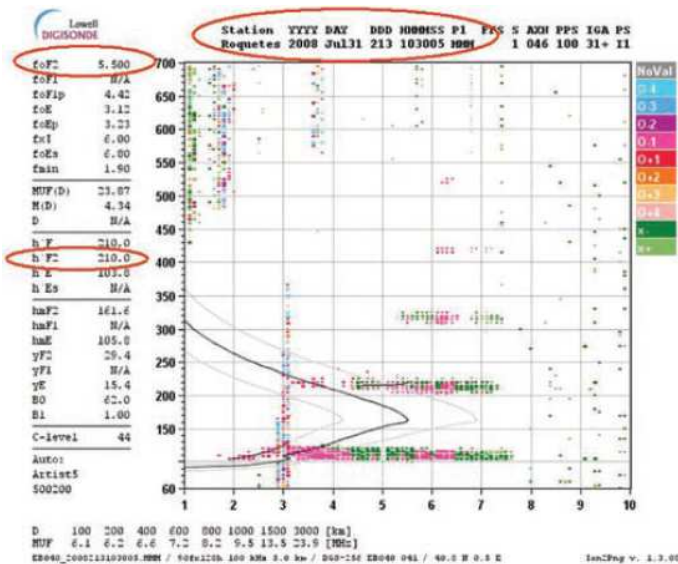
Figura 3: extracción de la frecuencia crítica foF2 de un ionograma
