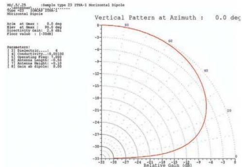
Figura 7: dipolo ubicado a un décimo de longitud de onda del suelo
