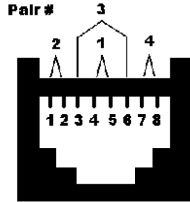
EIA/TIA 568B
