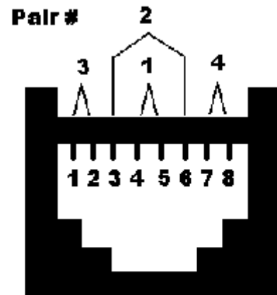
EIA/TIA 568A
